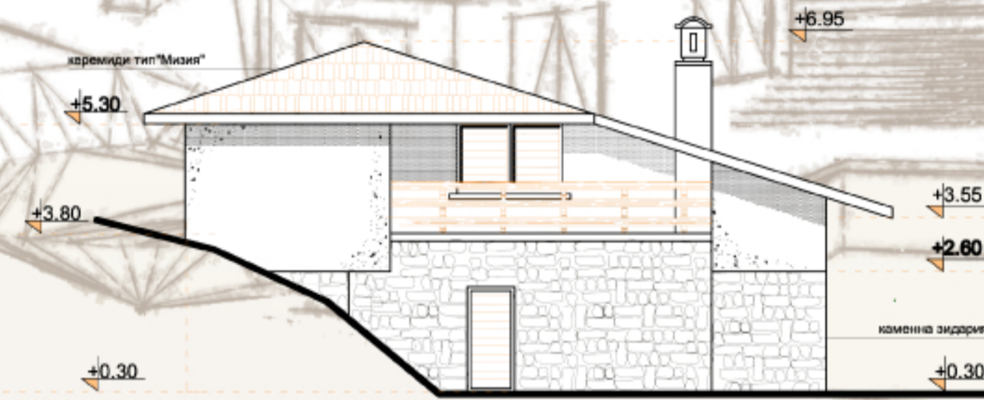
ФАСАДА СЕВЕРОЗАПАД М 1:100
