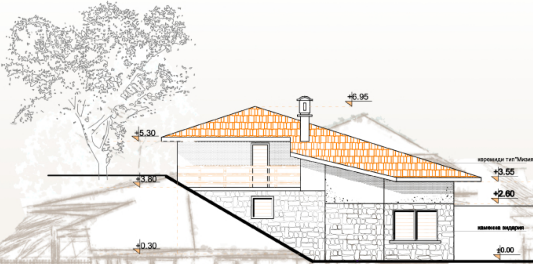
ФАСАДА ЮГОЗАПАД М 1:100
