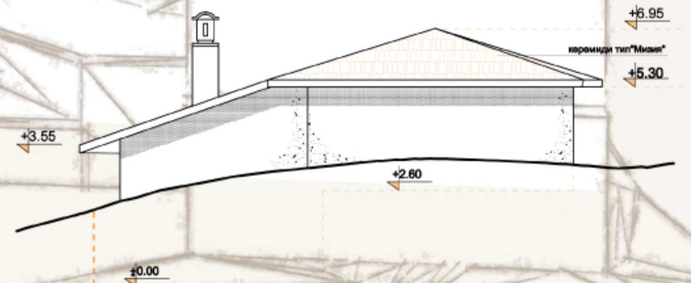
ФАСАДА СЕВЕРОИЗТОК М 1:100
