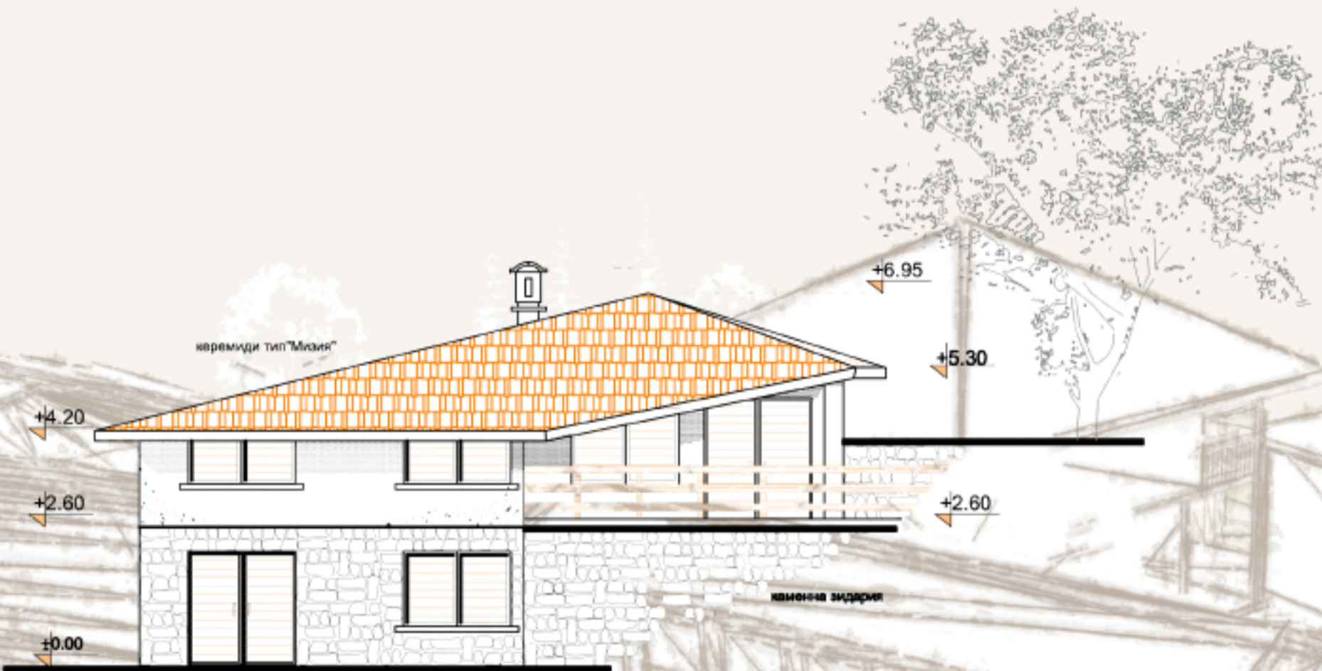
ФАСАДА ЮГОИЗТОК М 1:100
